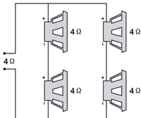
Последовательно-параллельное подключение
