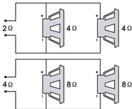
Параллельное подключение
