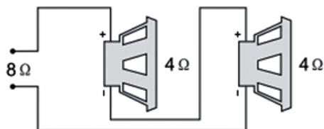
Последовательное подключение
